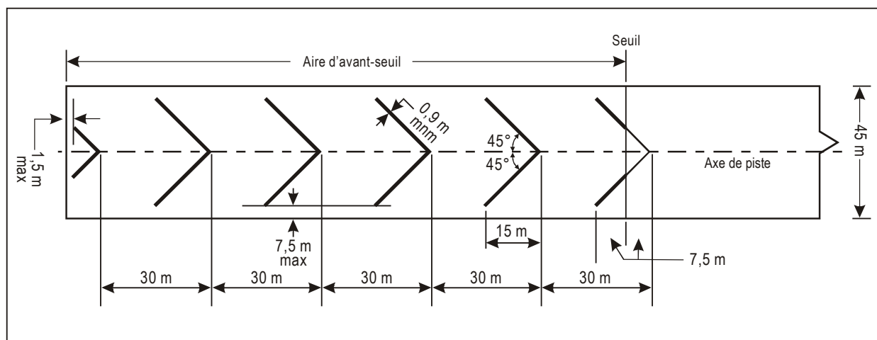
Figure 7-3. Marques d'avant-seuil
