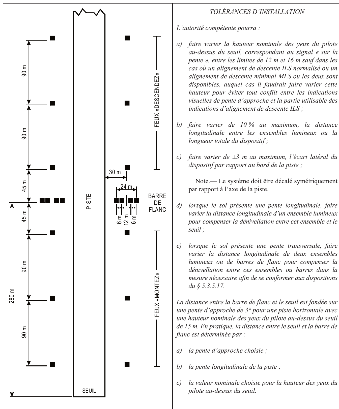
Figure 5-17. Emplacement des ensembles lumineux du T-VASIS
