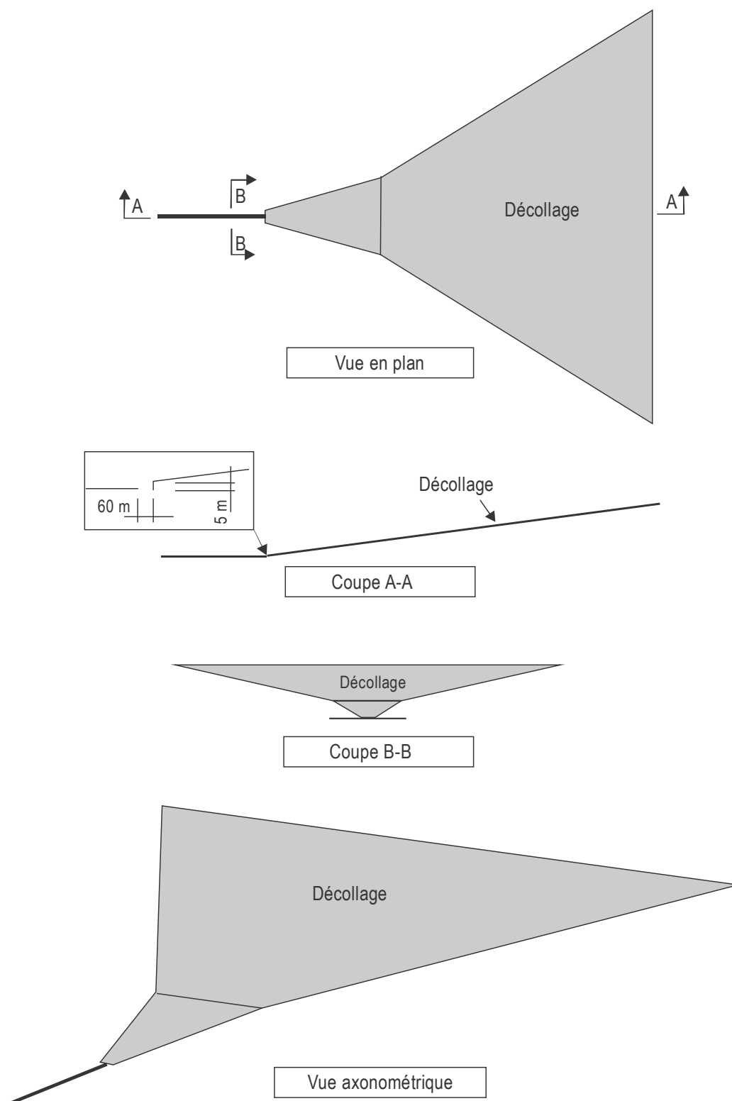
Figure 4-7. Surface de départ aux instruments
