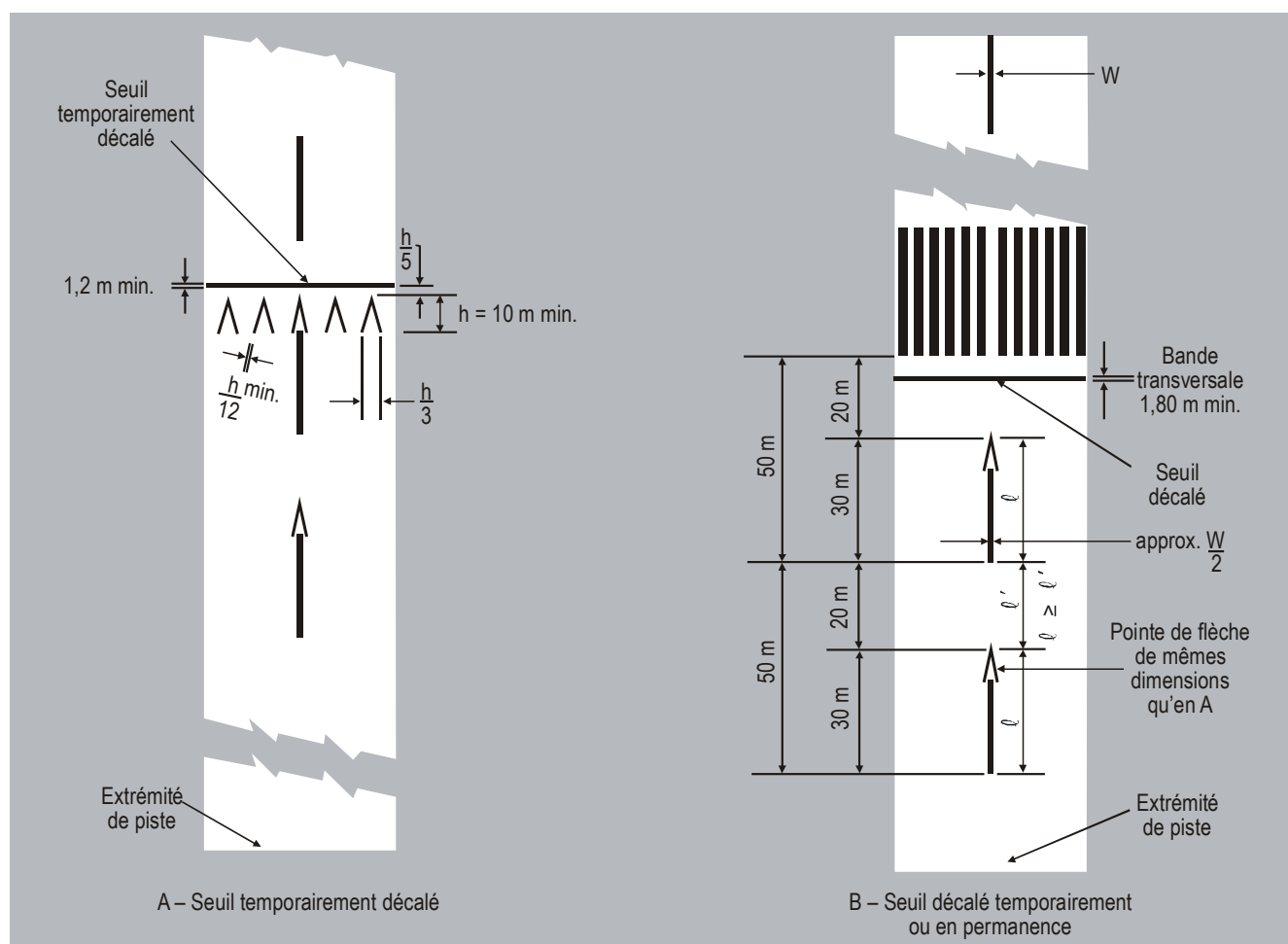
Figure 5-4. Marques de seuil décalé
