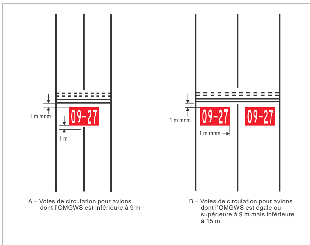
Figure 5-10. Marque d'obligation
