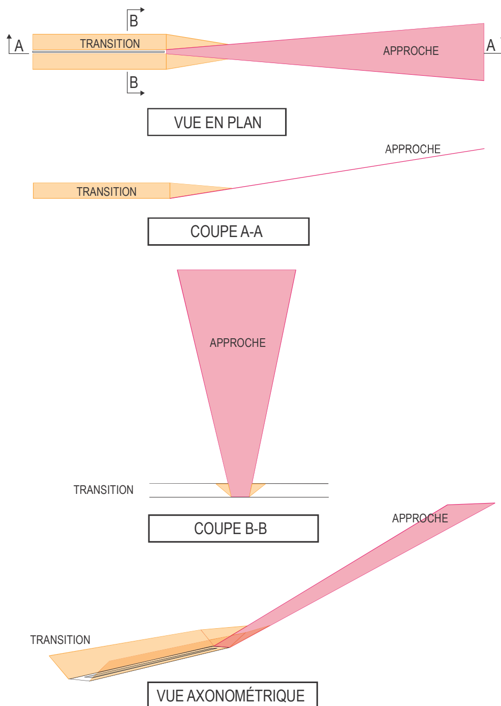
Figure 4-1. Surface d'approche et surfaces de transition
