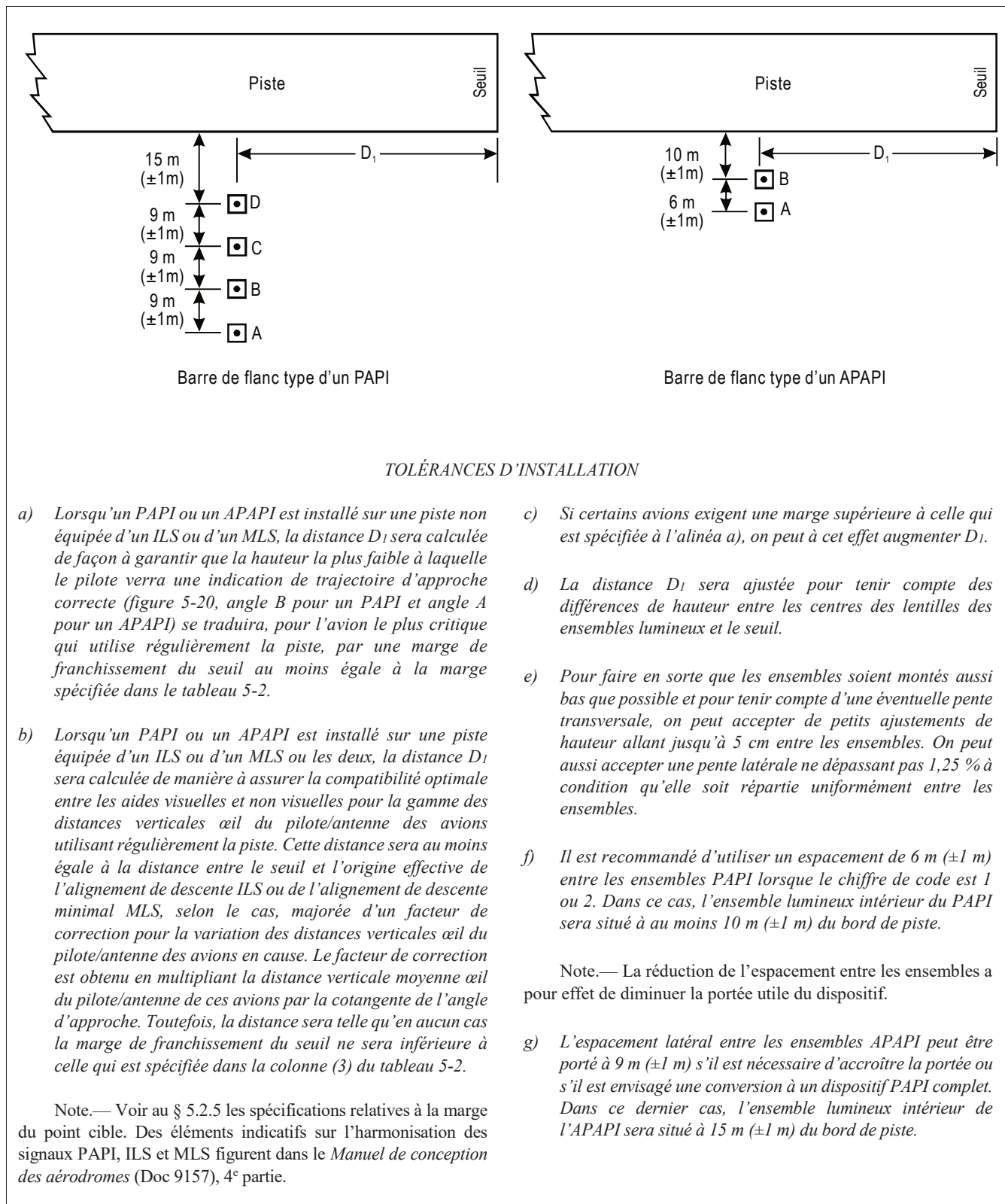
Figure 5-19. Implantation du PAPI et de l'APAPI
