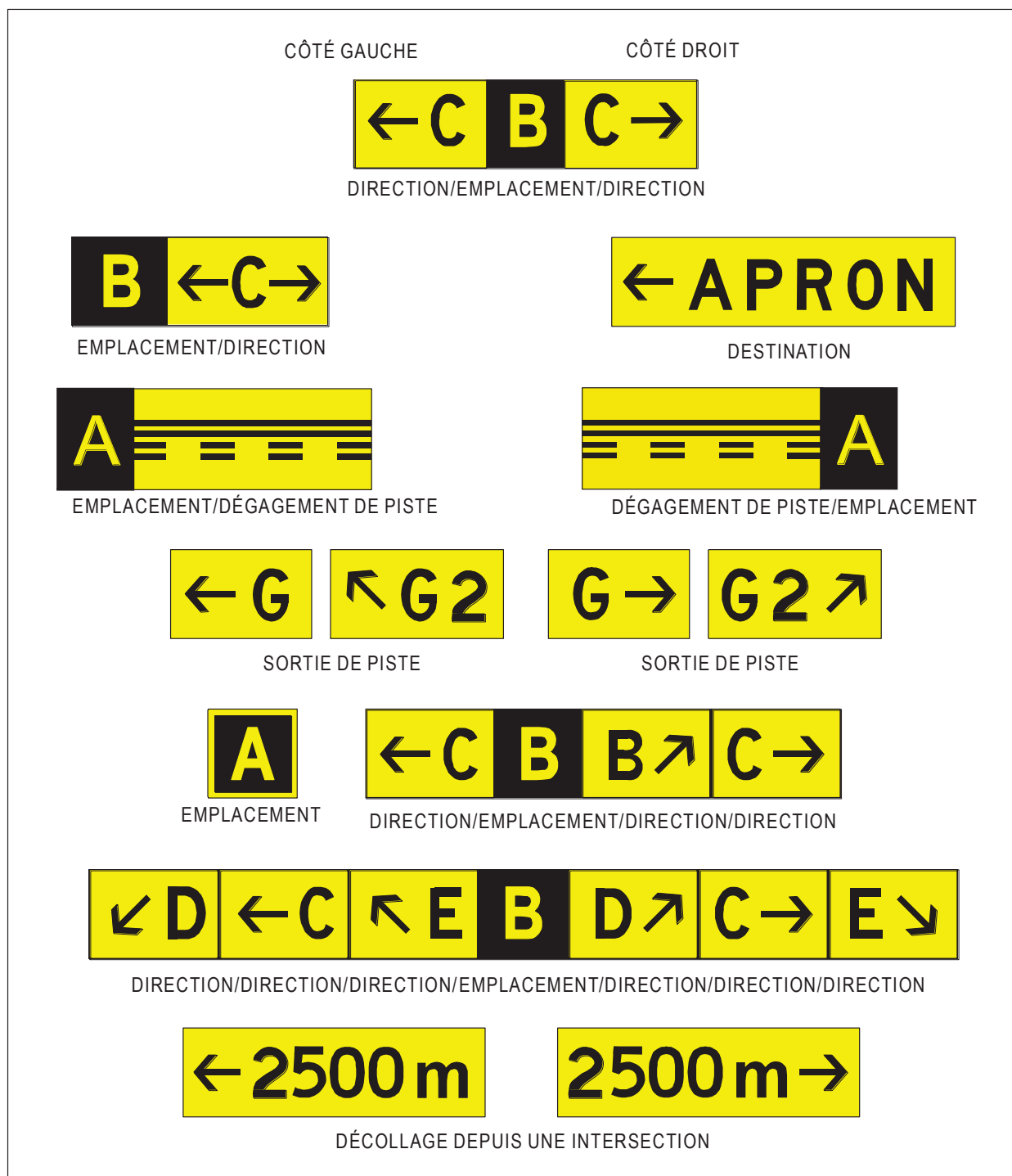
Figure 5-31. Panneaux d'indication
