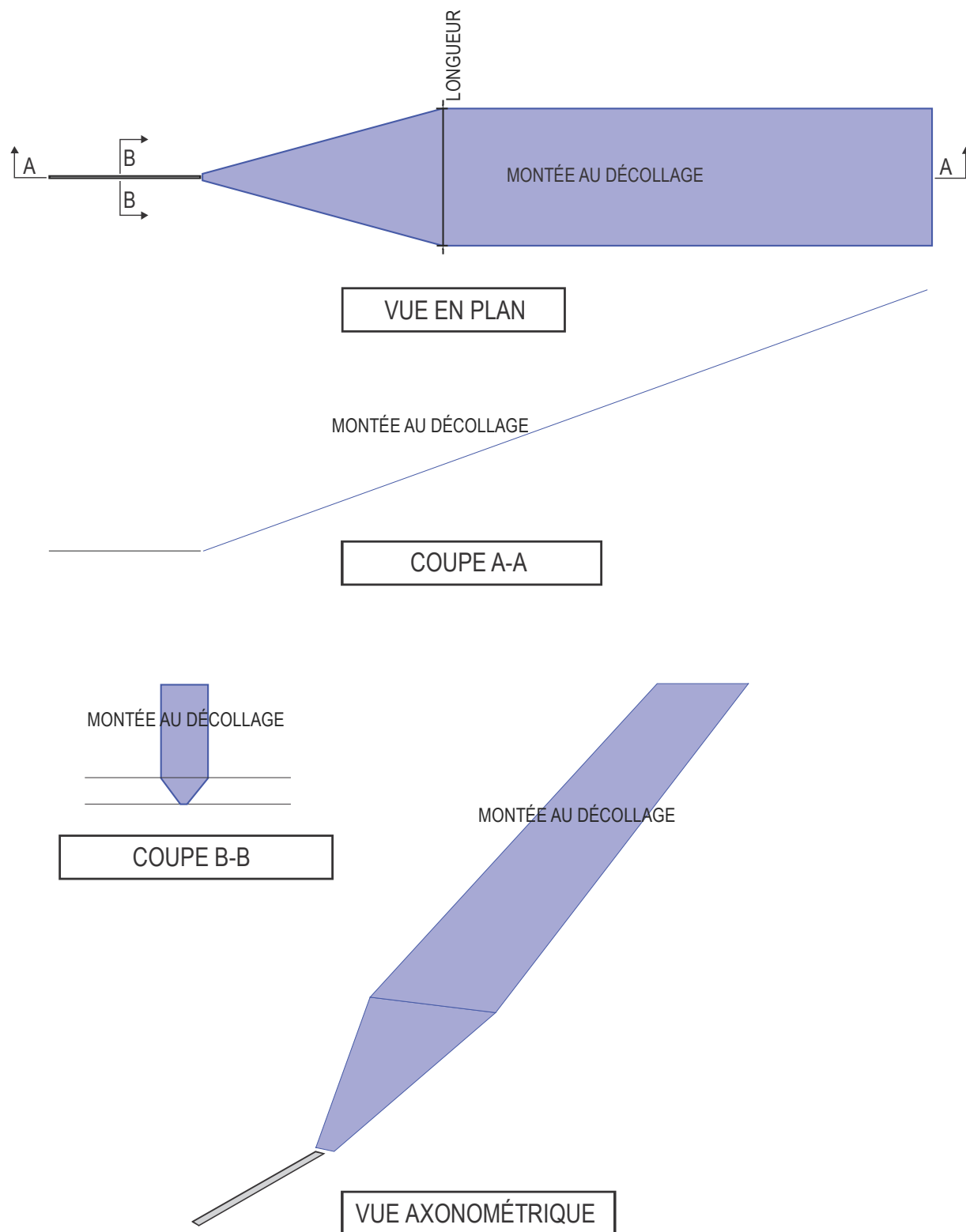
Figure 4-8 Surface de montée au décollage
