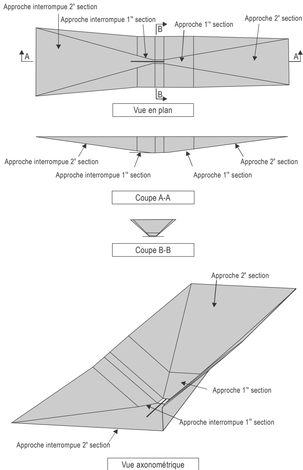
Figure 4-6. Surface pour approches de précision
