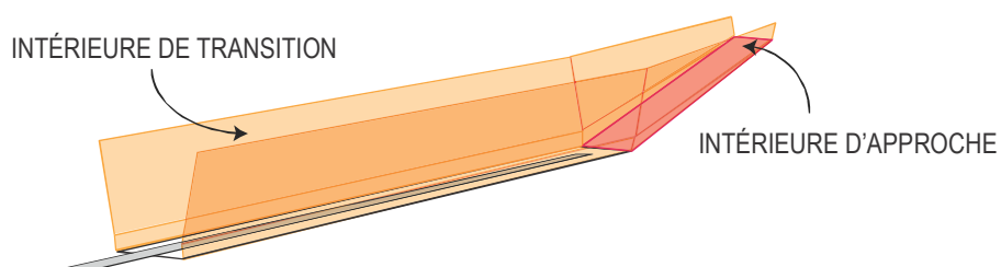
VUE AXONOMÉTRIQUE
