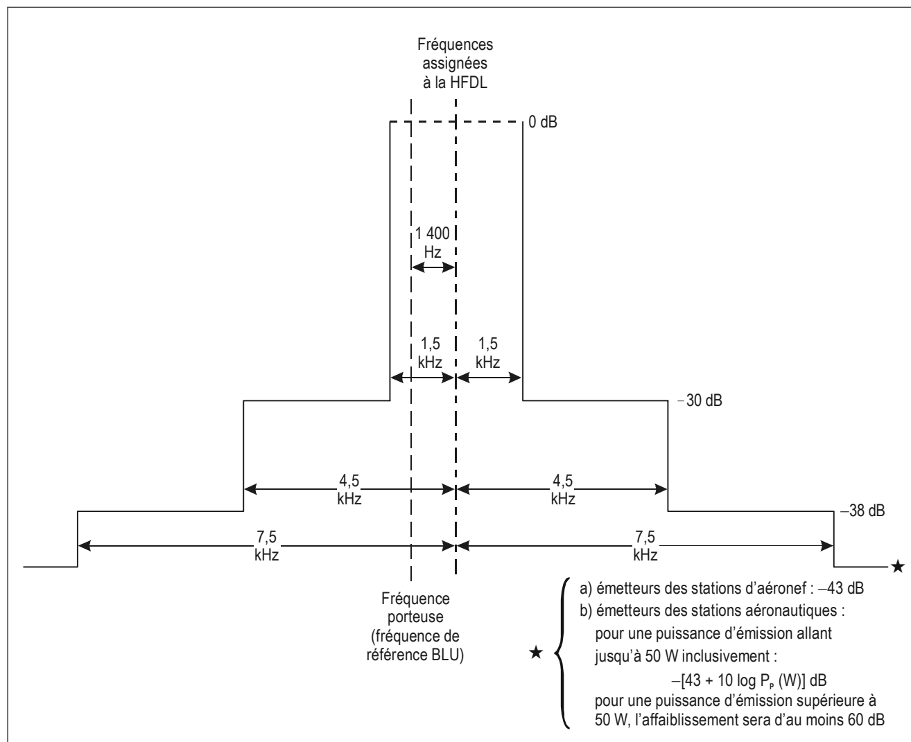
Figure 11-1. Limites spectrales requises (puissance de crête) pour les émetteurs des stations d'aéronef et des stations sol HFDF
