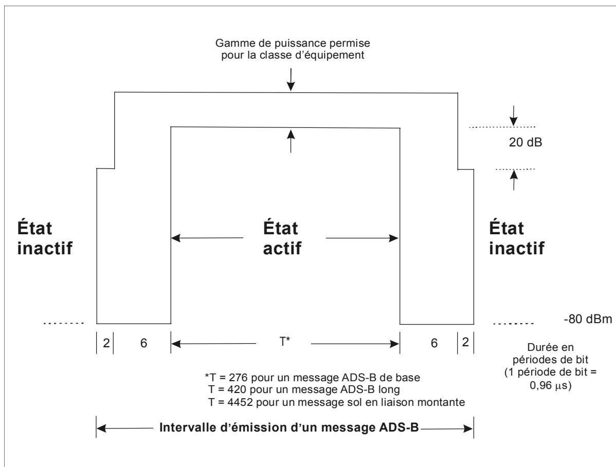
Figure 12-2. Profil temps-amplitude d'une émission d'un message UAT
