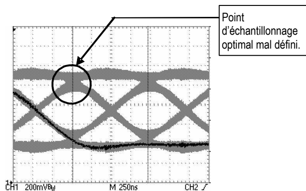
Figure 12-4. Diagramme en œil déformé
