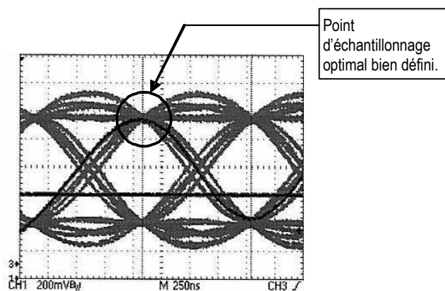
Figure 12-3. Diagramme en œil idéal
