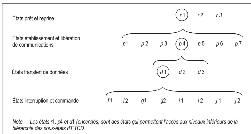
Figure 5-2. Hiérarchie des sous-états d'ETCD
