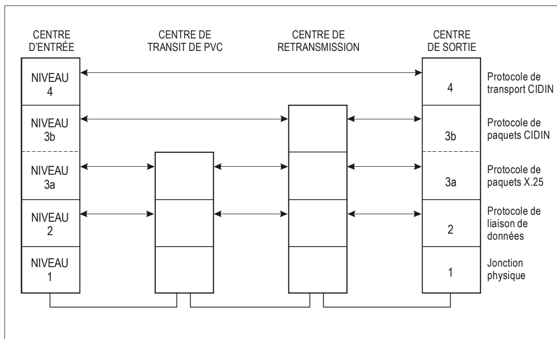
Figure 8-1. Niveaux de protocole CIDIN
