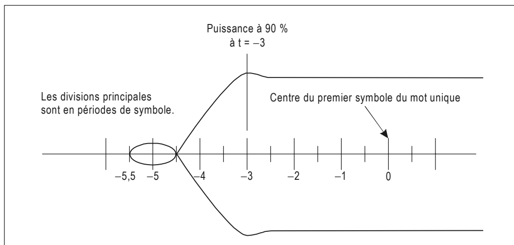
Figure 6-1. Stabilisation de la puissance de l'émetteur
